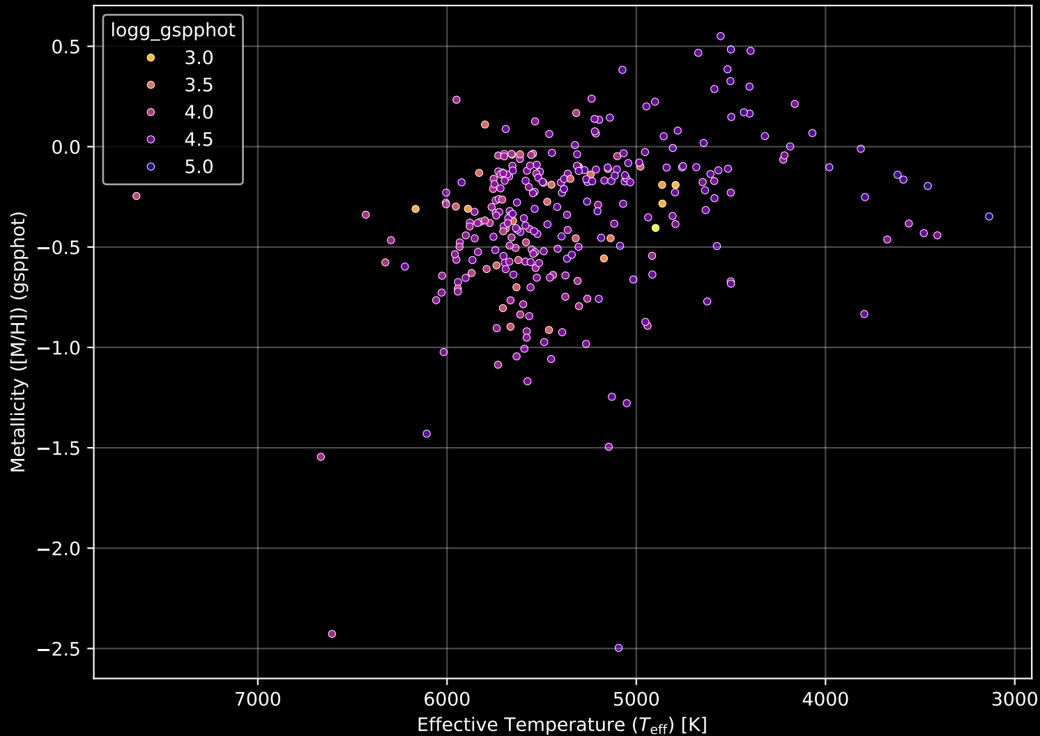
GALAH DR4 Field: [6690] Stellar Population Parameters (n= 289)
