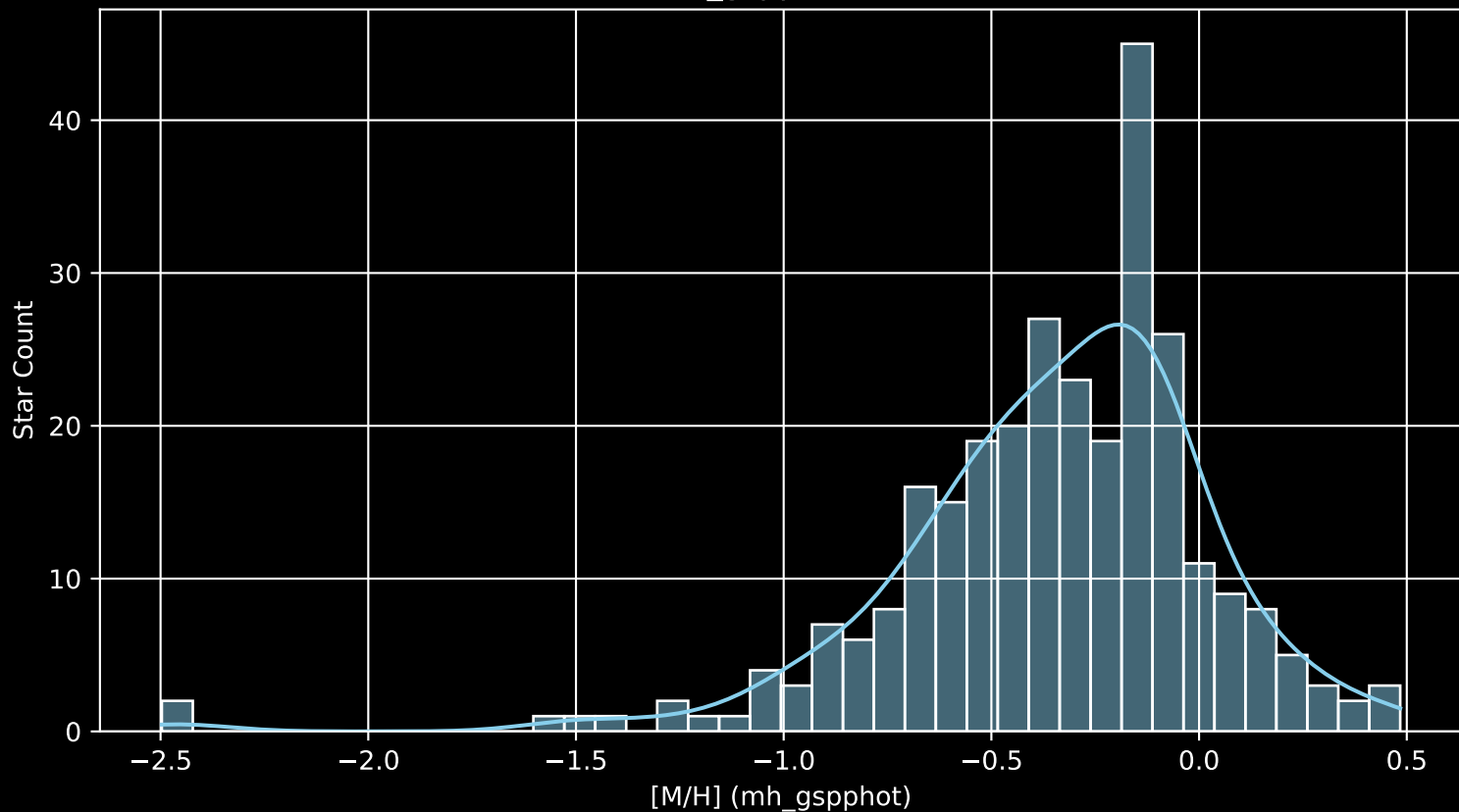
GALAH DR4 Field: [6690] [M/H] (mh_gspphot) (n= 288)
