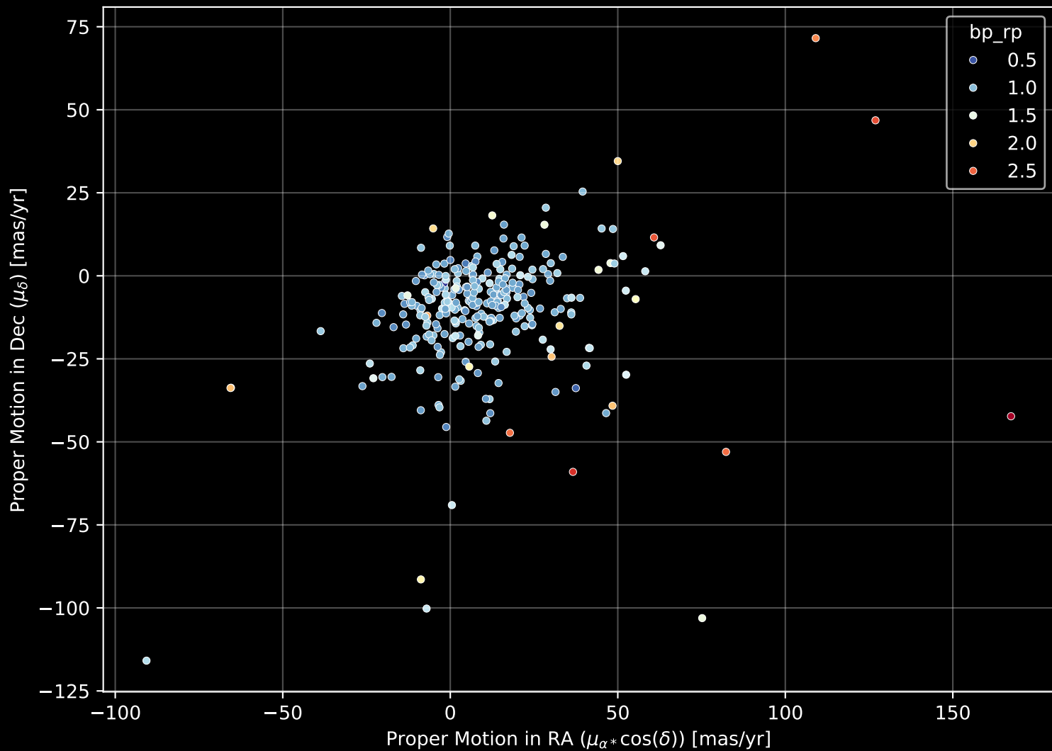
GALAH DR4 Field: [6690] Proper Motion Diagram (n= 289)
