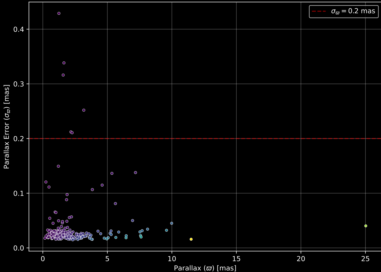
GALAH DR4 Field: [6690] Parallax Quality (n= 289)
